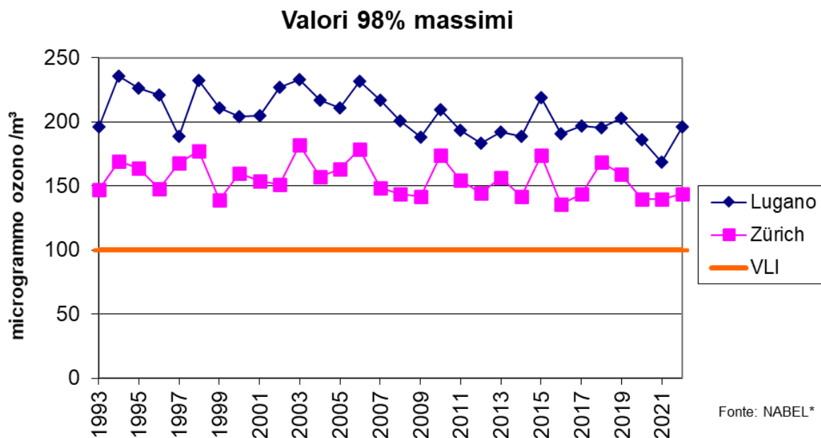
Fig. 1: L'inquinamento causato da elevate concentrazioni di ozono è descritto dal valore 98° percentile mensile massimo della media semioraria.
