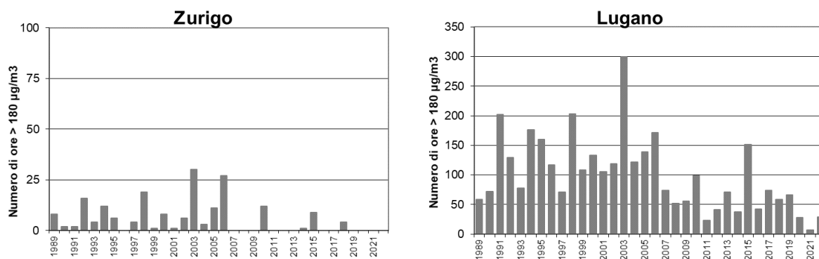
Fig. 3: Superamento del valore medio orario di 180 \mu\text{g}/\text{m}^3 a Zurigo e Lugano 1989-2022 (Fonte: NABEL).
